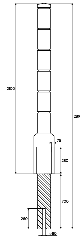
Размеры: 170*170*2810 (мм), рабочая высота 2100 (мм)
