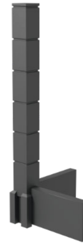
Размеры: 170*170*2810 (мм), рабочая высота 2100 (мм)
