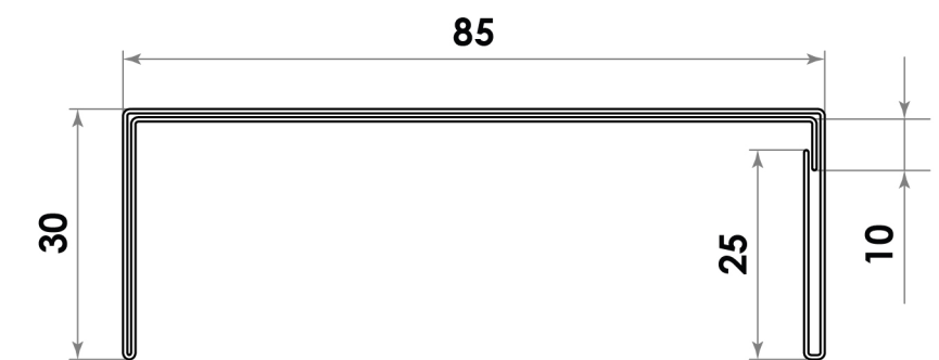
Планка для крепежа боковая
