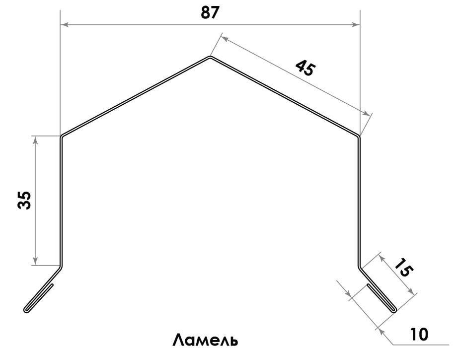
Верхняя заглушка
