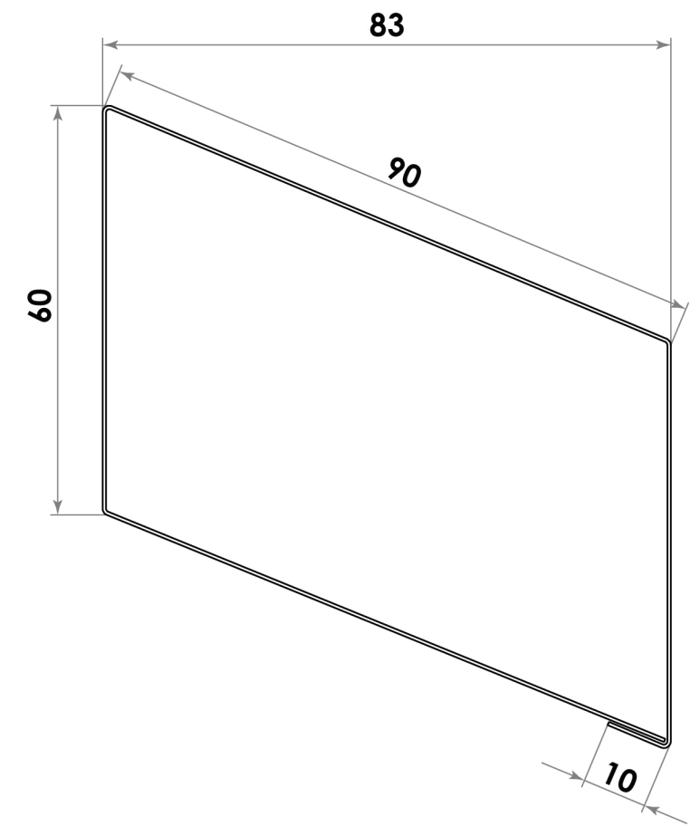
Планка для крепежа боковая
